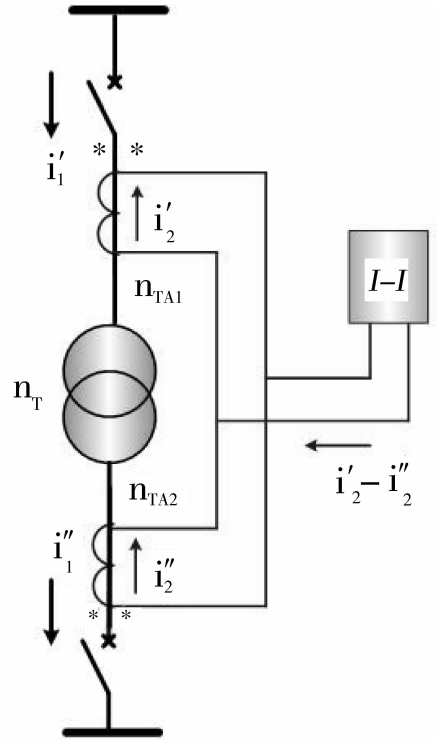
图 1 变压器纵差动保护原理接线图
