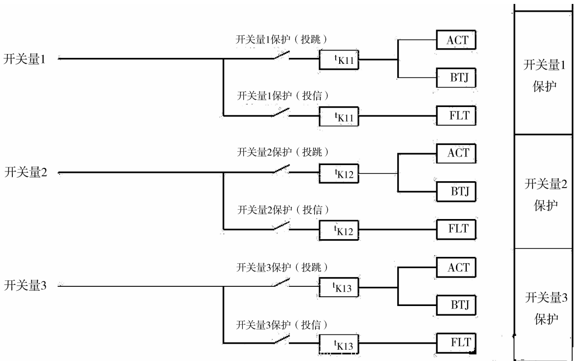
图 2 变压器非电量保护原理
