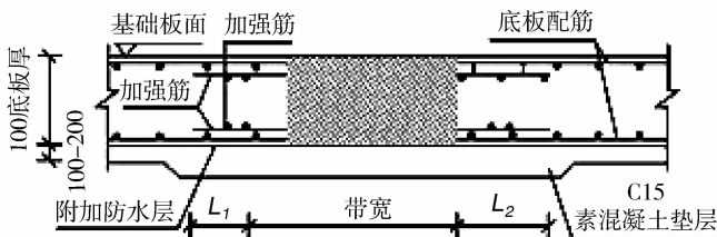
图4 底板及外墙后浇带
