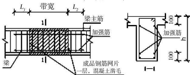
图3 主次梁后浇带构造要求
