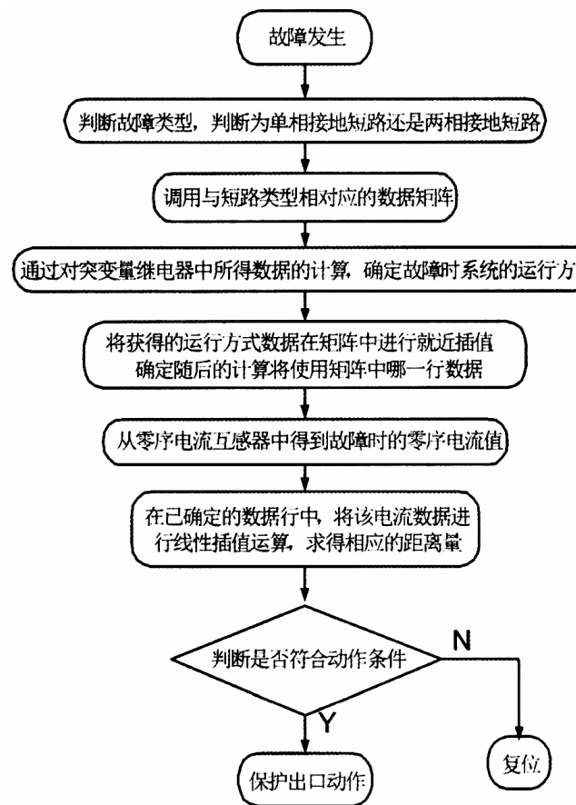
图 2 保护算法的计算流程图
