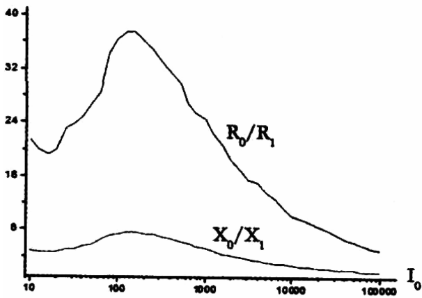
图 1 电缆零序电阻、电抗比和零序电流之间的关系曲线图
