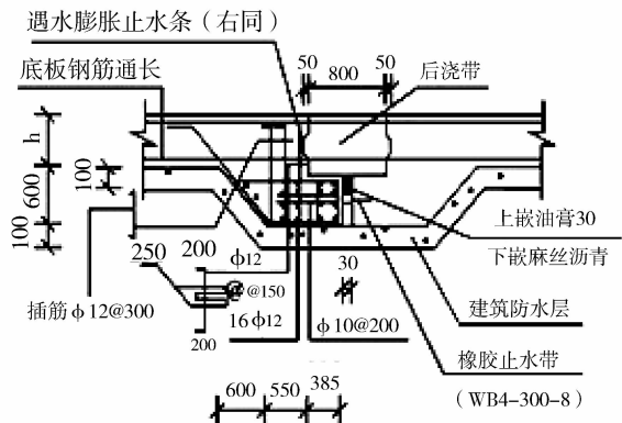
图1 地下室底板后浇带的施工和构造
