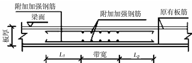
图2 楼板后浇带
